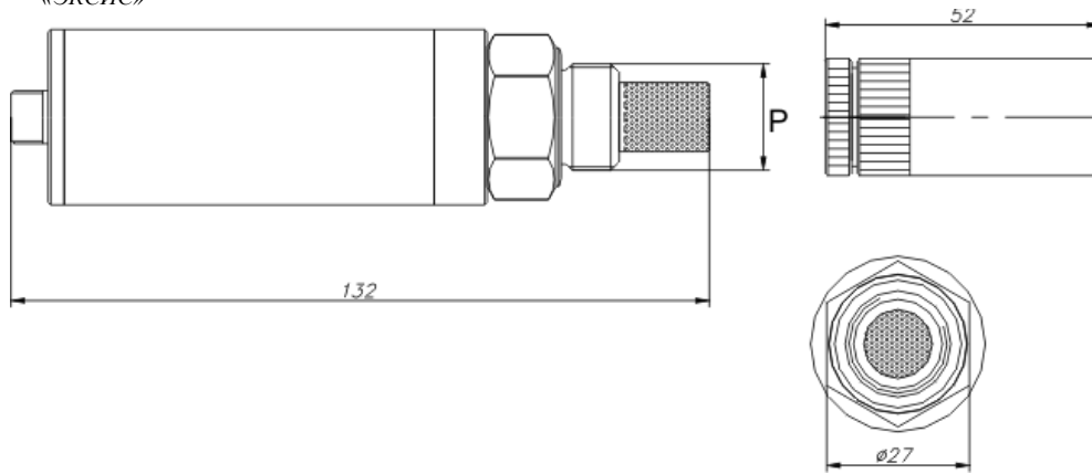
Рисунок 3.4 Внешний вид измерительного преобразователя ИПВТ-08
